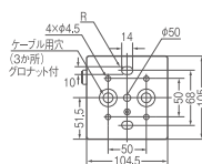
取付金具
