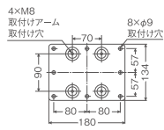
取付け台
