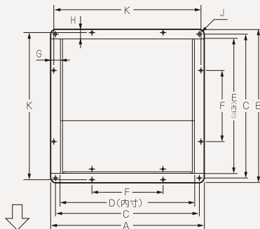
■ 寸法図 SCFF - 25-30-35-40-50-60-75-90
