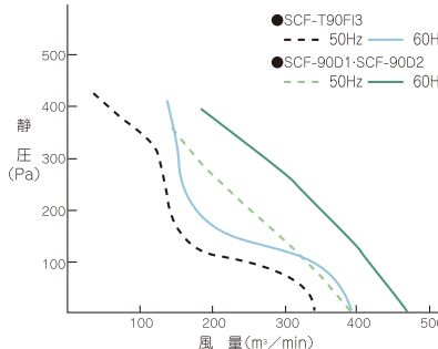
■ SCF-T90FI3 (標準型3相200V) ■ SCF-90D1 (耐圧防爆型3相200V) ■ SCF-90D2 (安全増防爆型3相200V)
